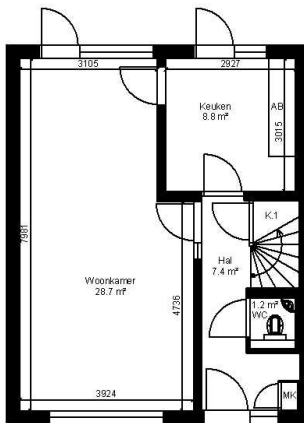
Begane grond
