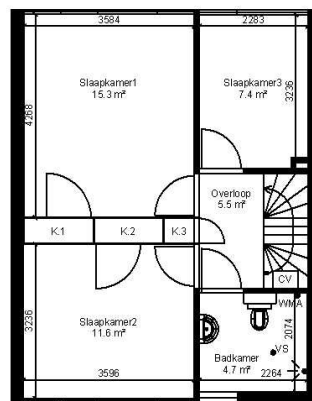
Verdieping
