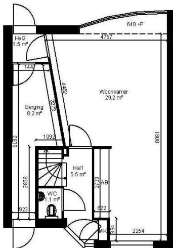
Begane grond
